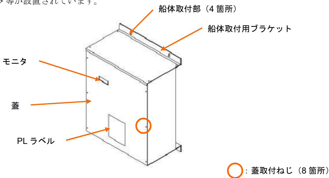
図 2-7 モータドライバ本体の外観形状
