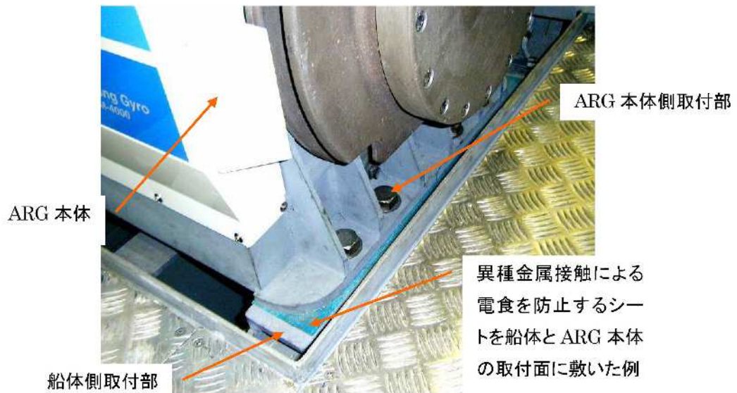
図 4-5 ARG 本体の取付面における電食防止処理の例
