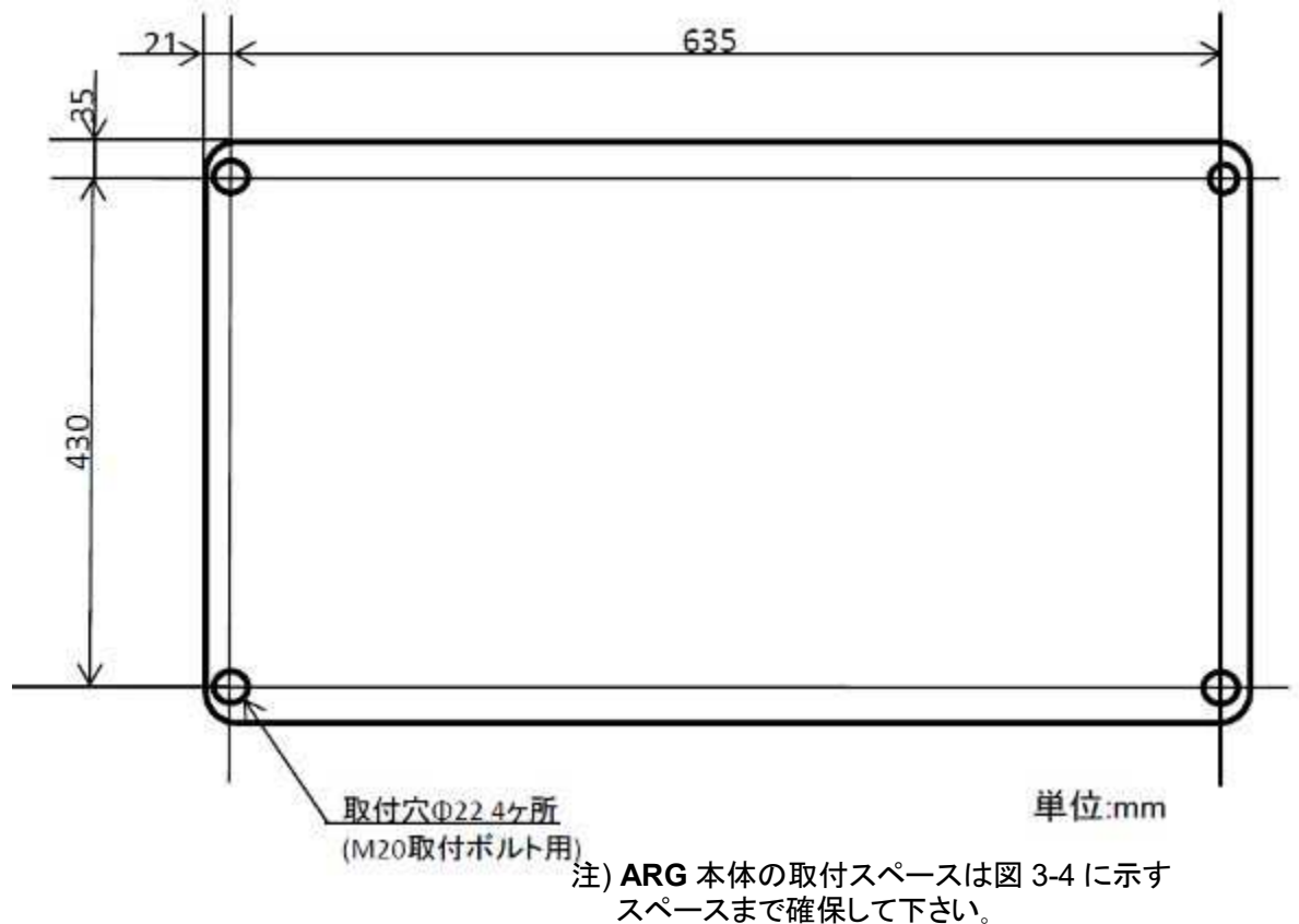
図 4-1 ARG 本体の取付穴寸法
