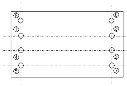
図 4-7 ボルトの締付順序 (例)
