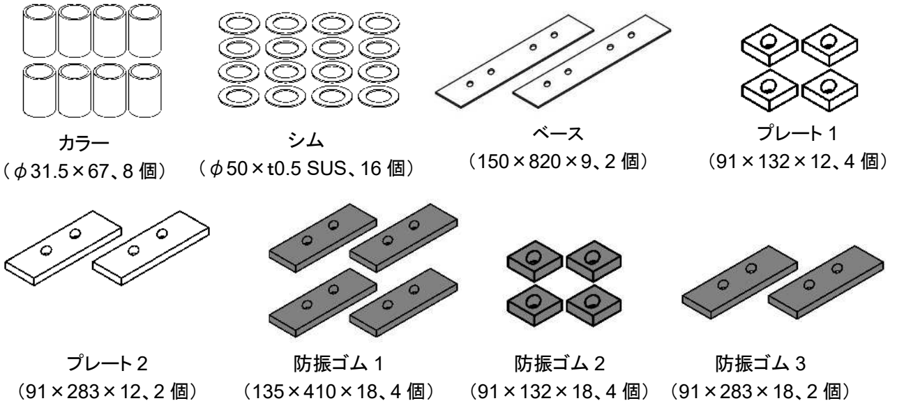
図 2-2 梱包箱の中味の確認 (その 2)
