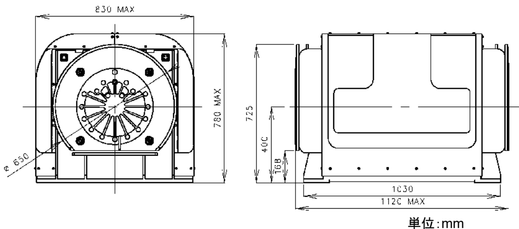
図 2-6 ARG 本体の寸法
