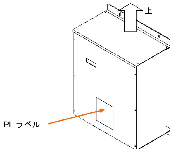
図 4-9 モータドライバの取付方向
