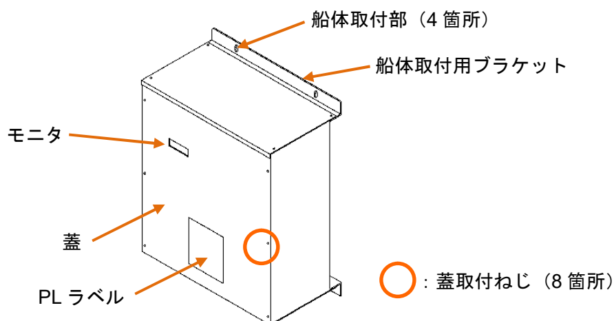
図 2-8 モータドライバ本体の外観形状
