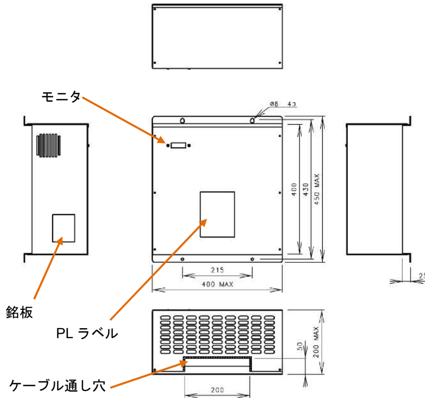
図 2-9 モータドライバの寸法
