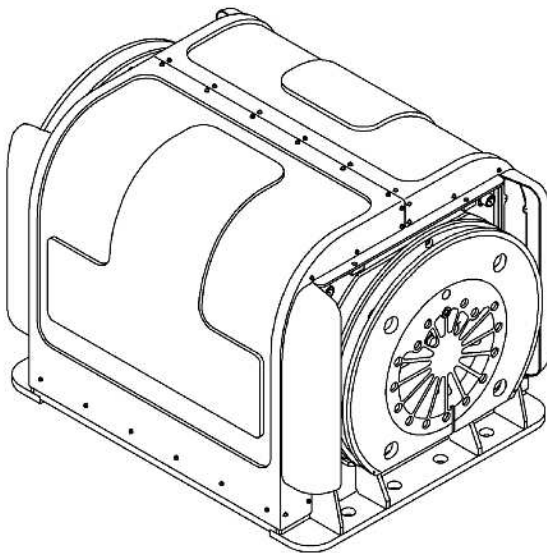
ARG 本体 (MSM-37500T-A1、1 台)
