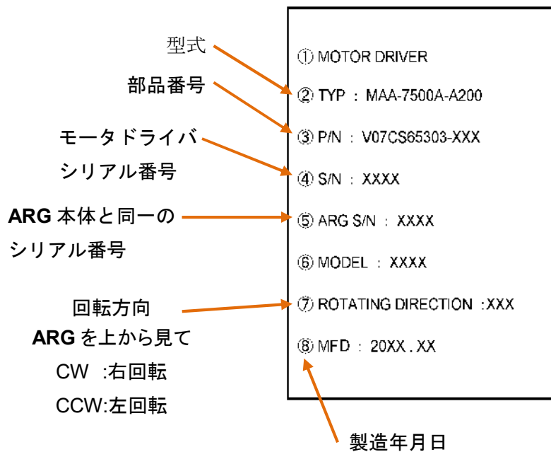
図 2-10 モータドライバの銘板
